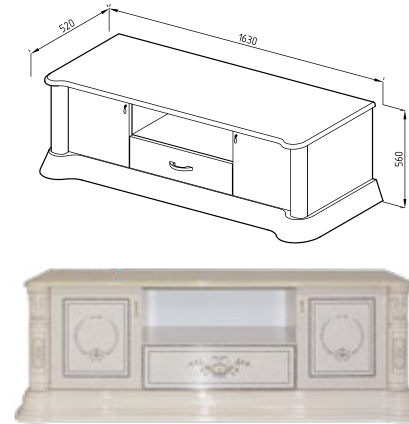
ТВ-тумба / TV-closet д/л | в/н | г/д 1630 | 560 | 520
