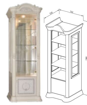
Вітрина 1Д / Vitrine 1D д/л | в/н | г/д 740 | 2180 | 520
